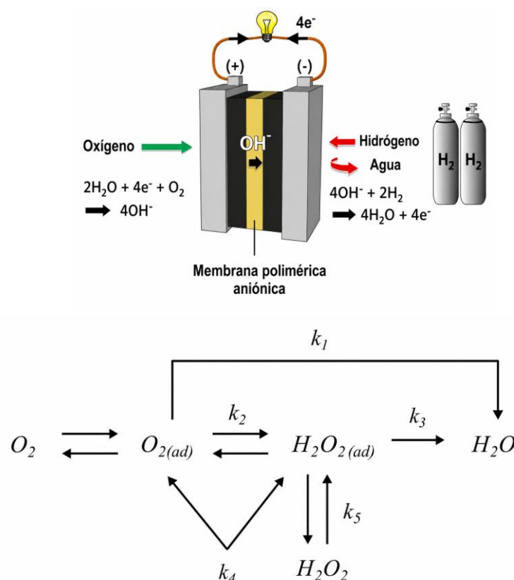
Figura 8. Pila de combustible PEM con las reacciones que tienen lugar en sus electrodos (arriba) y mecanismo general para la ORR en medio ácido (abajo) con la vía de 4 electrones a \text{H}_2\text{O} y de 2 electrones a \text{H}_2\text{O}_2 .
