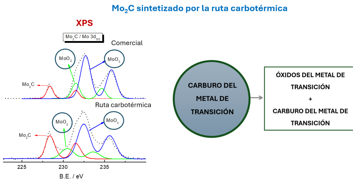
Figura 16. Caracterización por XPS mostrando la presencia de óxido de molibdeno en la superficie del carburo, tanto del sintetizado como del comercial. (García et al., 2016).
